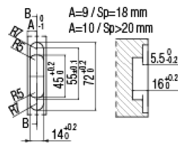
Mecanismo fecho de porta móvel de cozinha.
