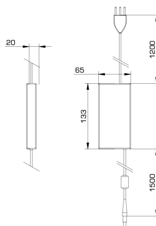
TRANSFORMADOR
