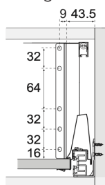
Montagem Traseira
