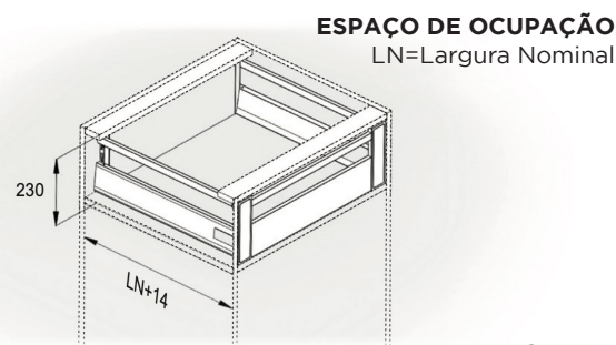
ESQUEMA
