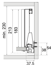
Montagem Traseira
