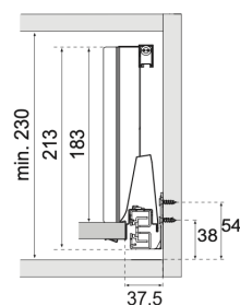
Montagem Traseira
