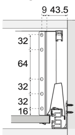
Montagem Traseira
