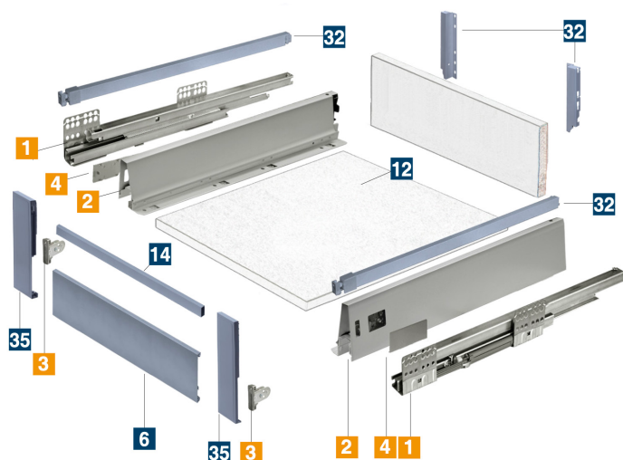
ESQUEMA
