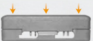
Posição correta: Pressionar com os três parafusos em paralelo
