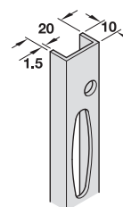
Largura do gancho
