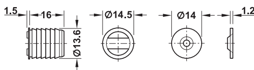
Caixa
