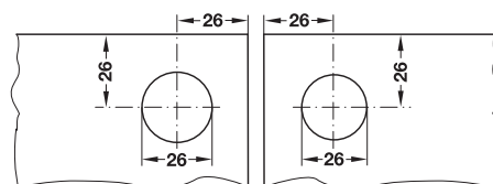
Padrão de furação para fechadura de palanca para portas de vidro, contrapeça
