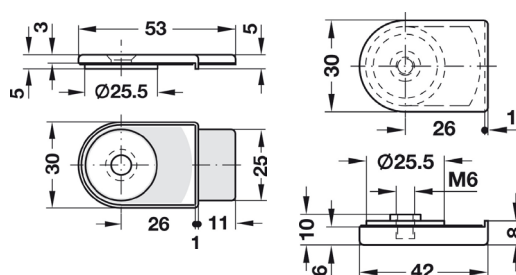
Padrão de furação para fechadura de palanca para portas de vidro, contrapeça
