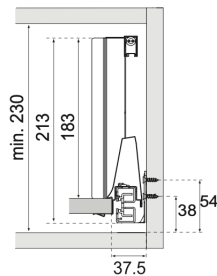
Montagem Traseira
