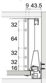
Montagem Traseira
