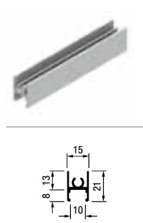
PERFIL SUPERIOR RS-BASE
