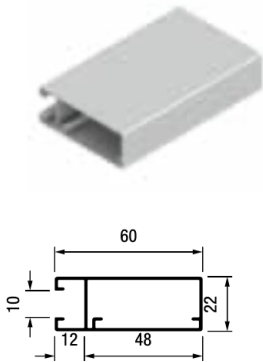
PERFIL PUXADOR TB 60
